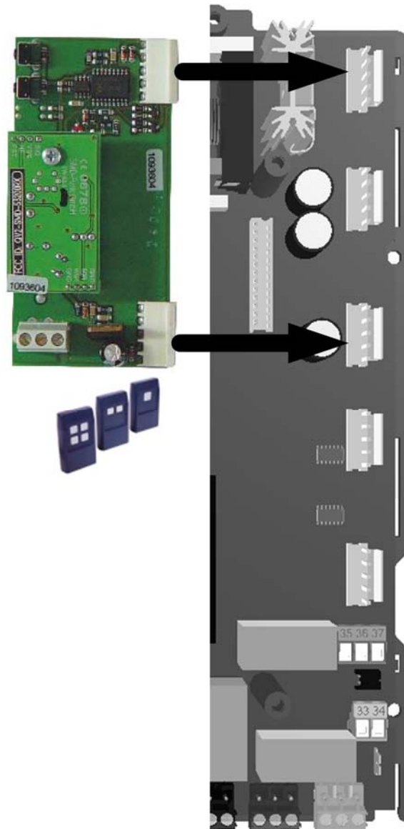
Abbildung 27: Funk-Steckempfänger
