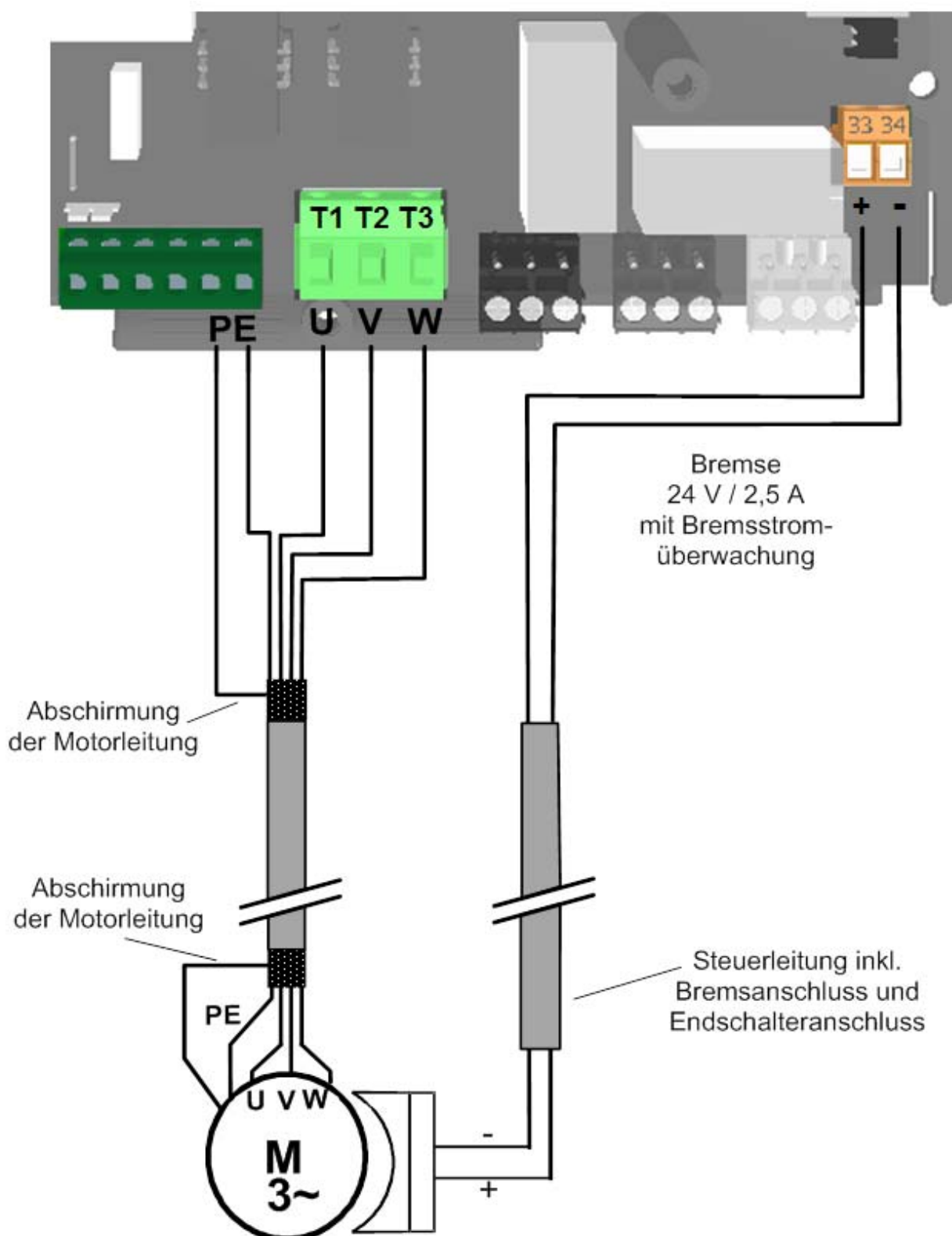
Abbildung 7: Motoranschluss mit 24 VDC Bremse
