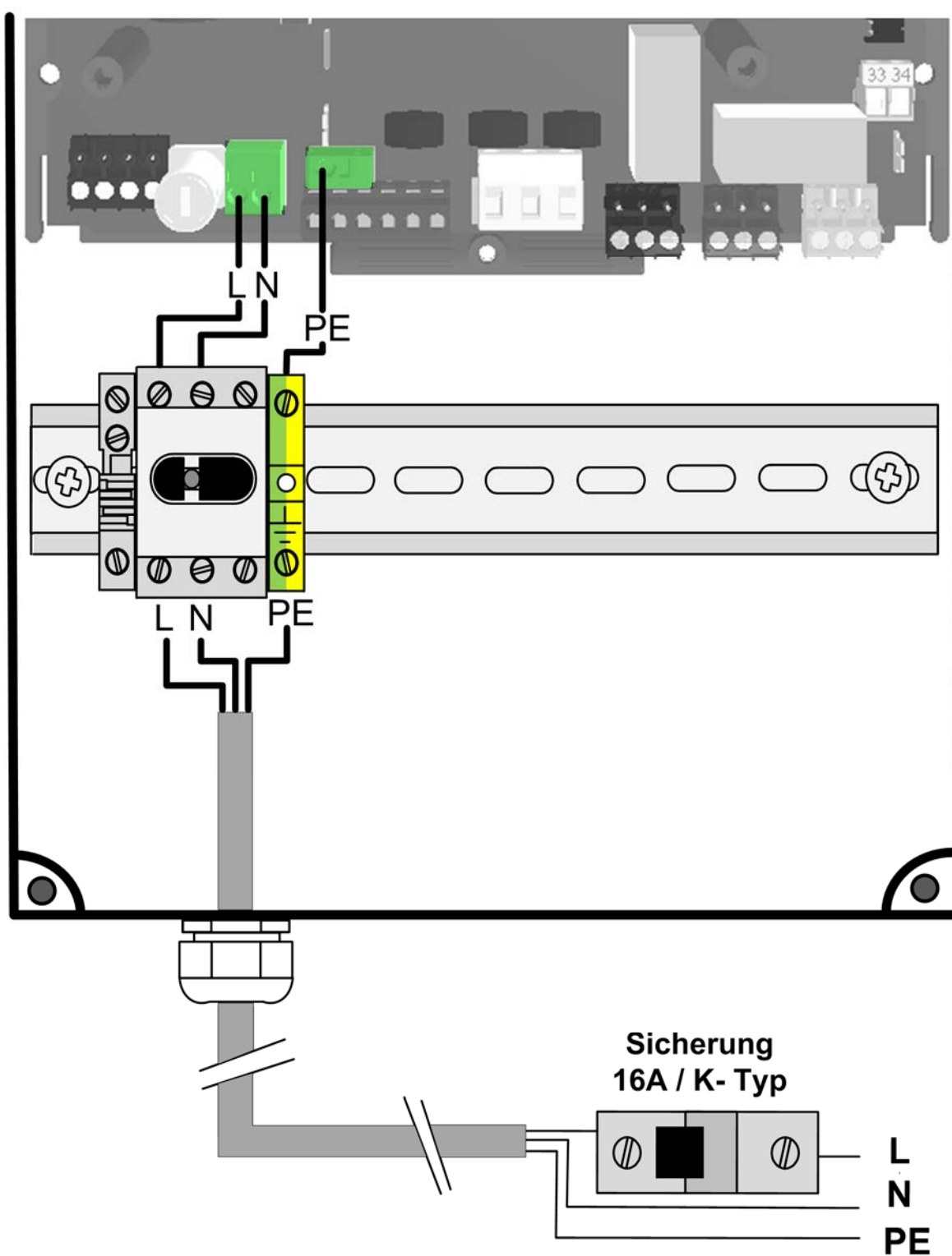
Abbildung 3: Anschluss Netzleitung
