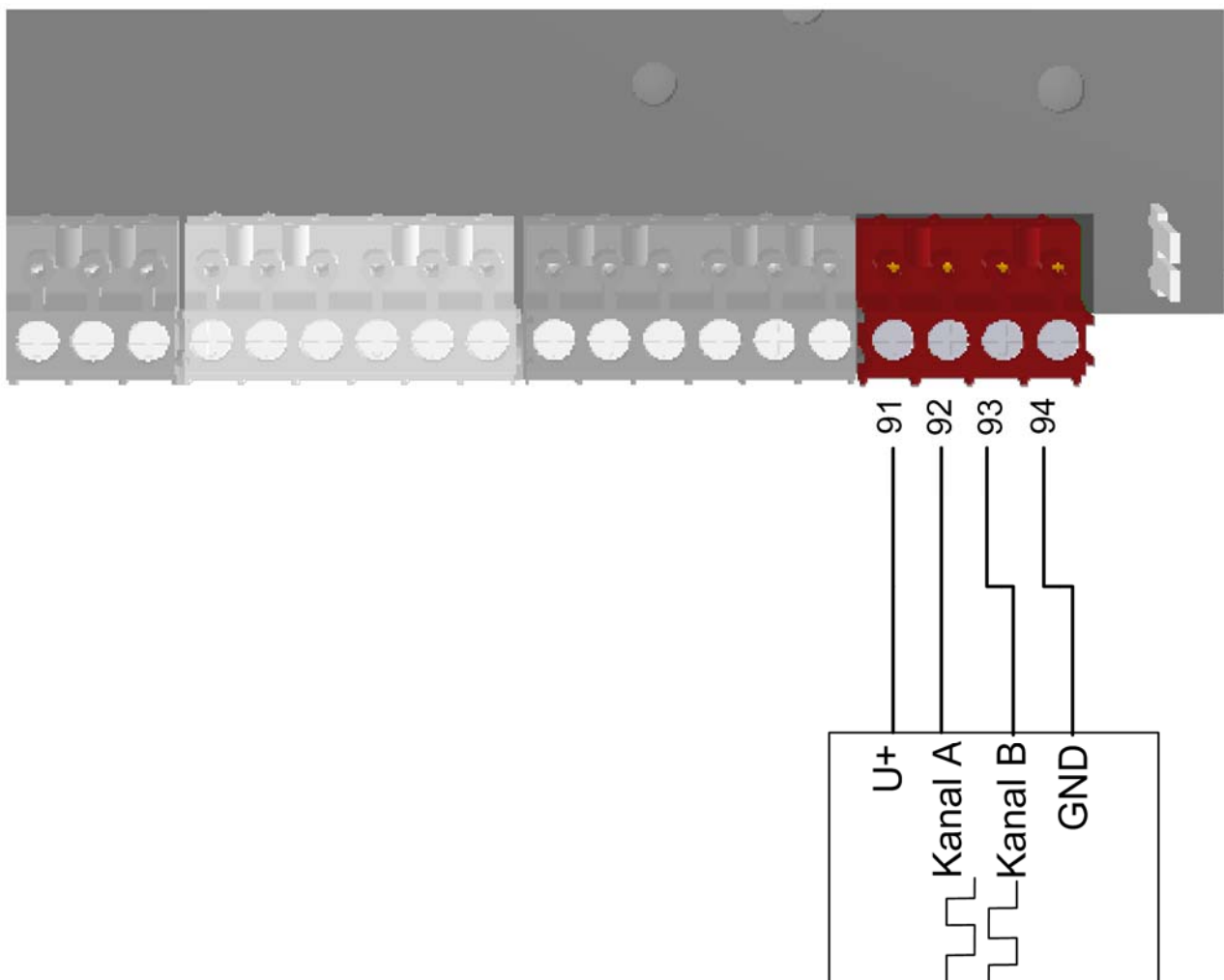
Abbildung 20: Anschluss Inkrementalgeber
