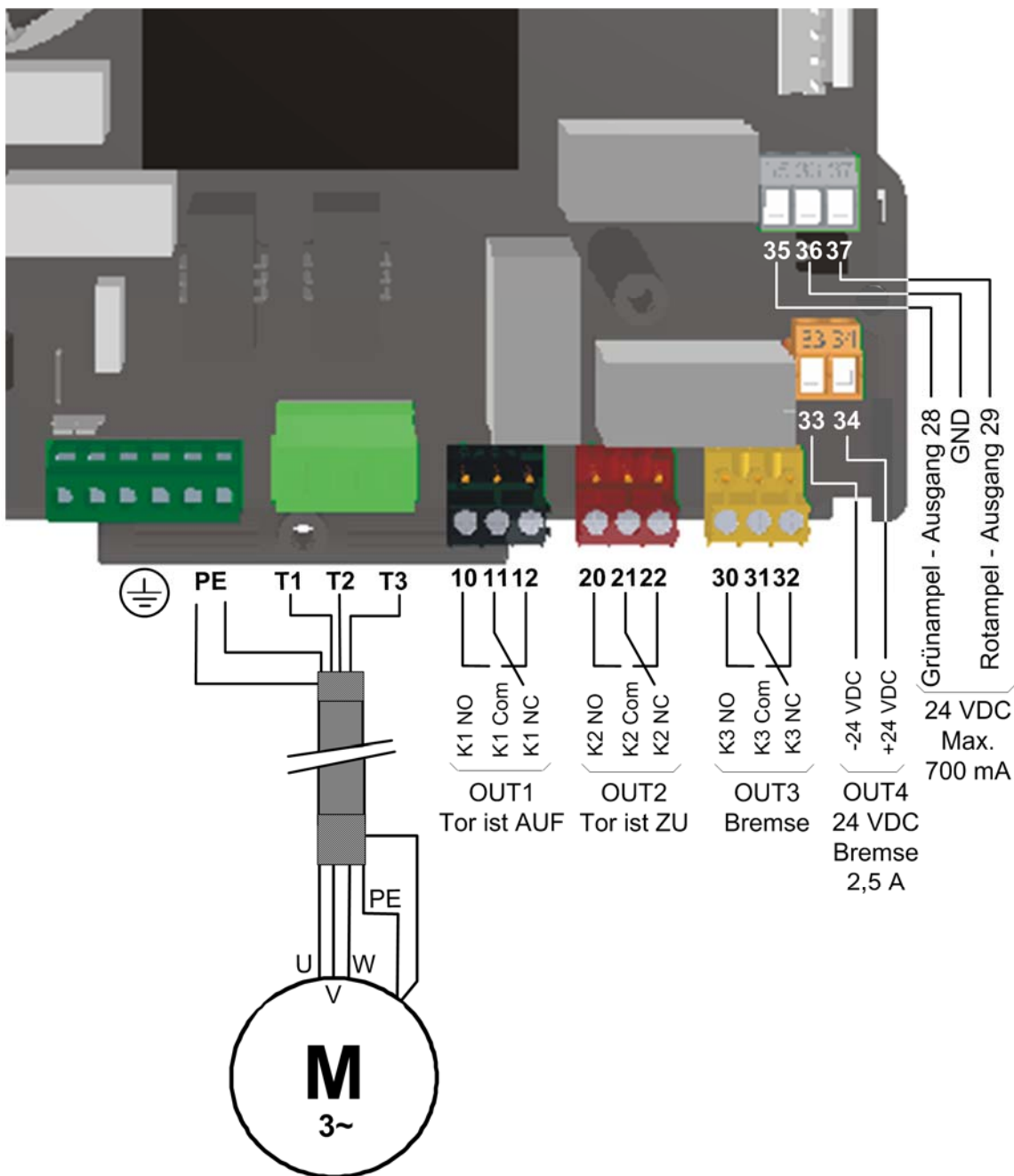
Abbildung 25: Übersicht Ausgänge
