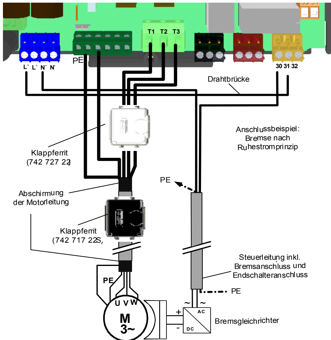
Abbildung 6: Motoranschluss
