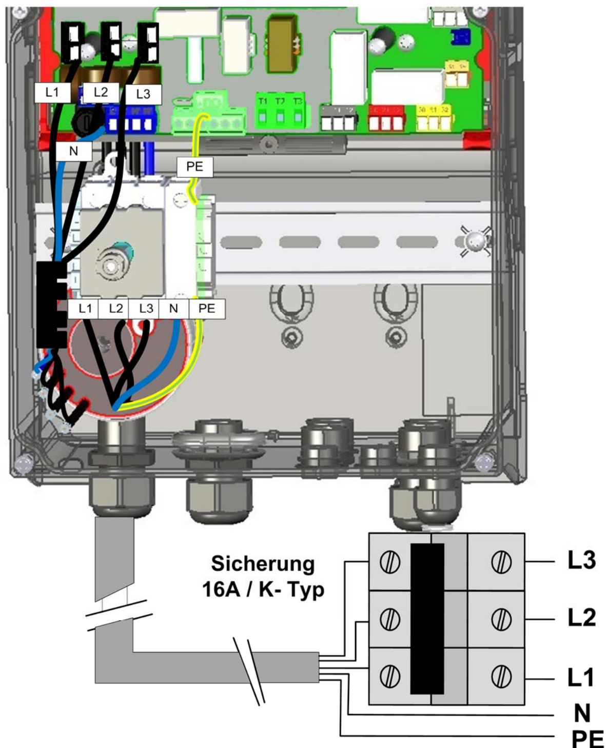
Abbildung 4: Anschluss Netzleitung
