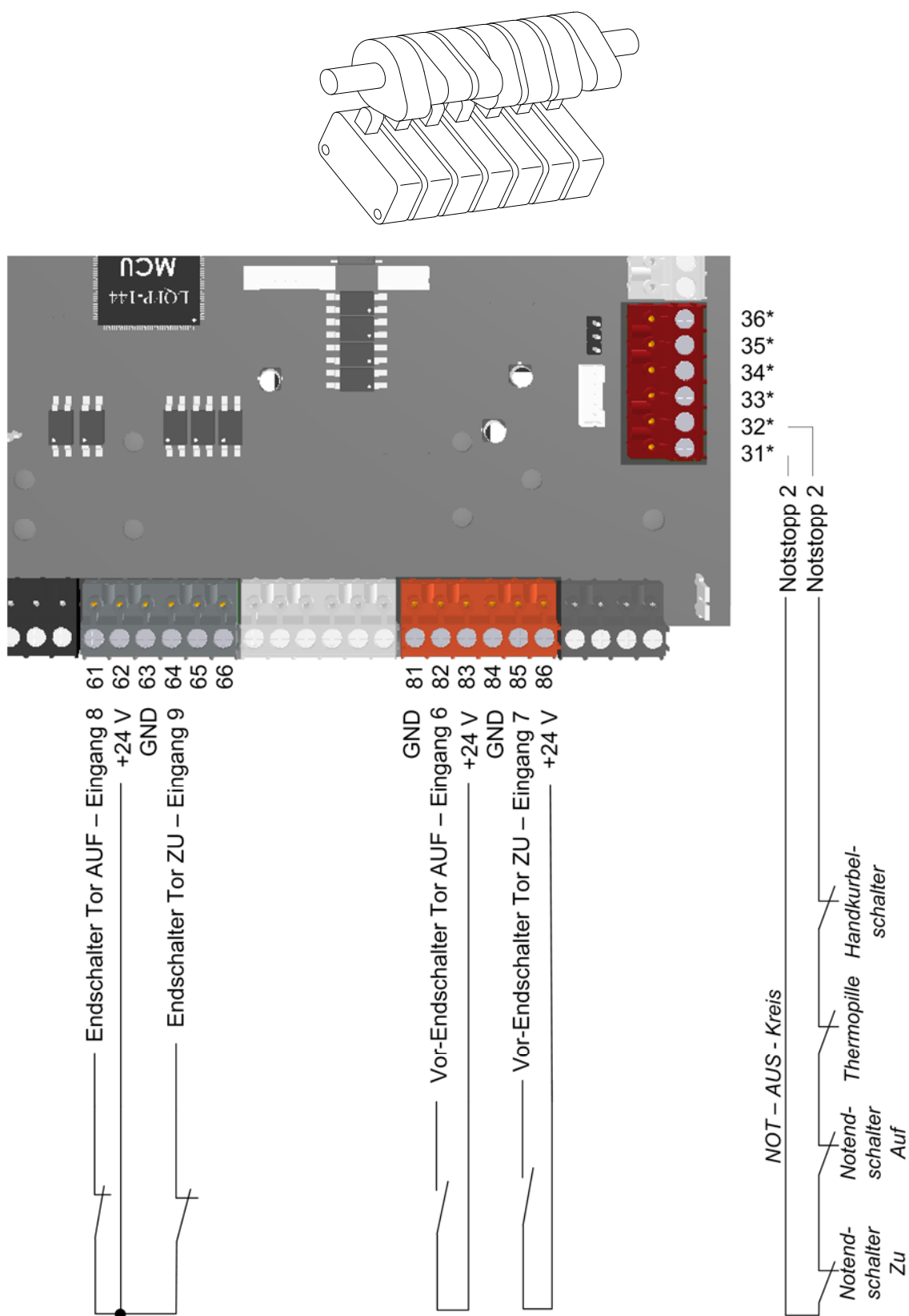
Abbildung 21: Anschluss Nockenendschalter
