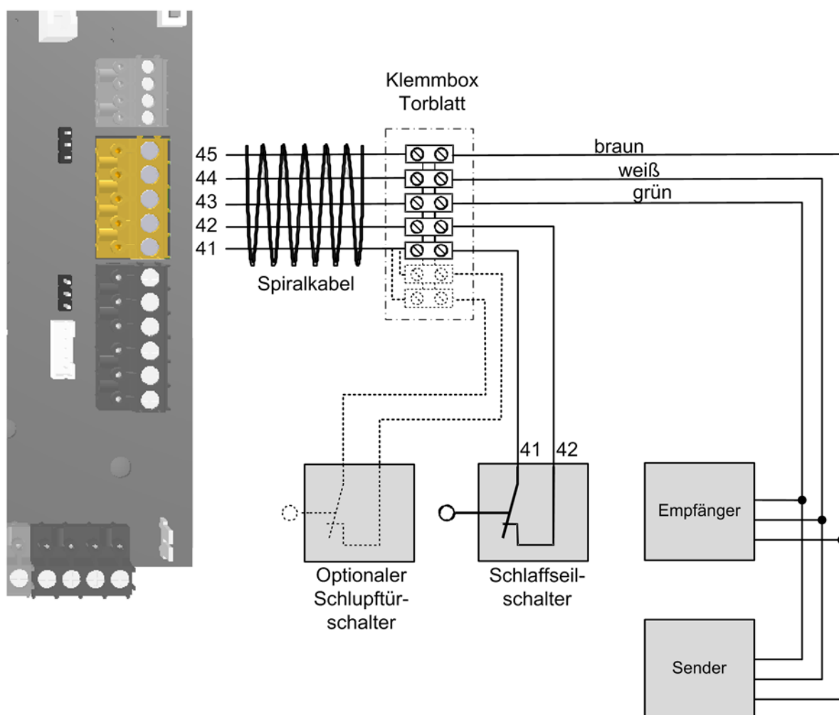
Abbildung 8: Anschluss einer optischen Sicherheitsleiste
