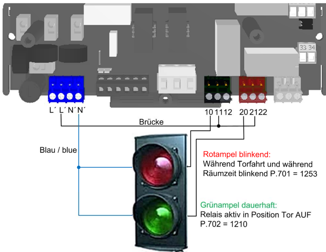
Abbildung 24: Ampelanschluss
