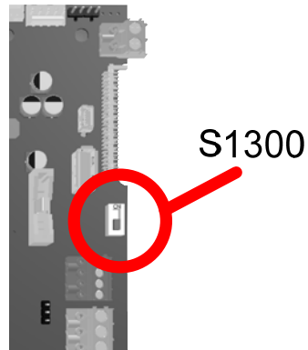
Abbildung 33: Position DIP- Schalter
